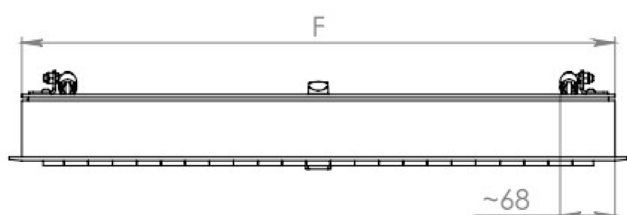
PRZEKRÓJ A-A SKALA 1 : 7
