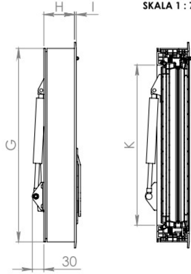
PRZEKRÓJ B-B SKALA 1 : 7
